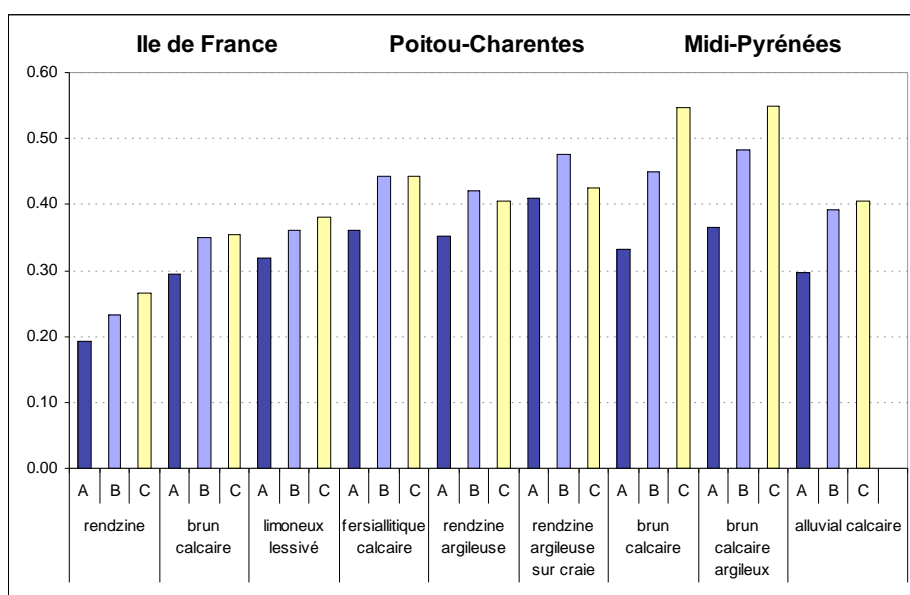
Figure A.2. Moyennes interannuelles de l'élévation de température de la surface agricole par rapport à l'air ( \Delta T en °C) par région, système de culture et sol
