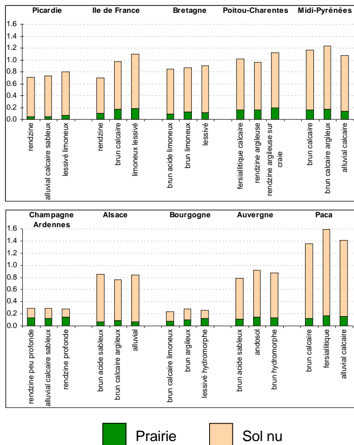
Figure 6. Ecarts moyens de température annuelle entre la surface et l'air (°C) par type de sol (en abscisse), les sols étant regroupés par région.
